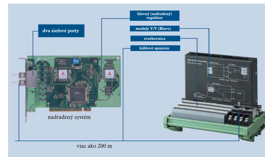
Schéma HSL
