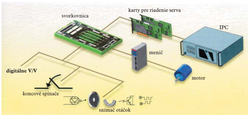
Schematické znázornenie riadenia motorov
